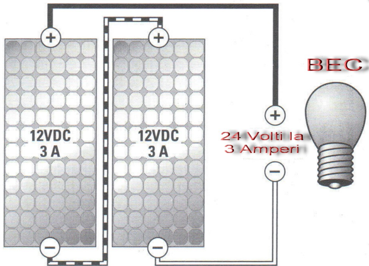
Panouri solare in serie
