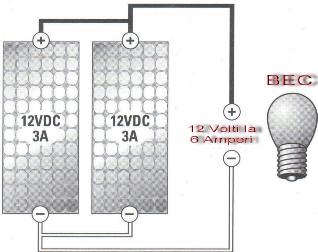
Panouri solare in paralel
