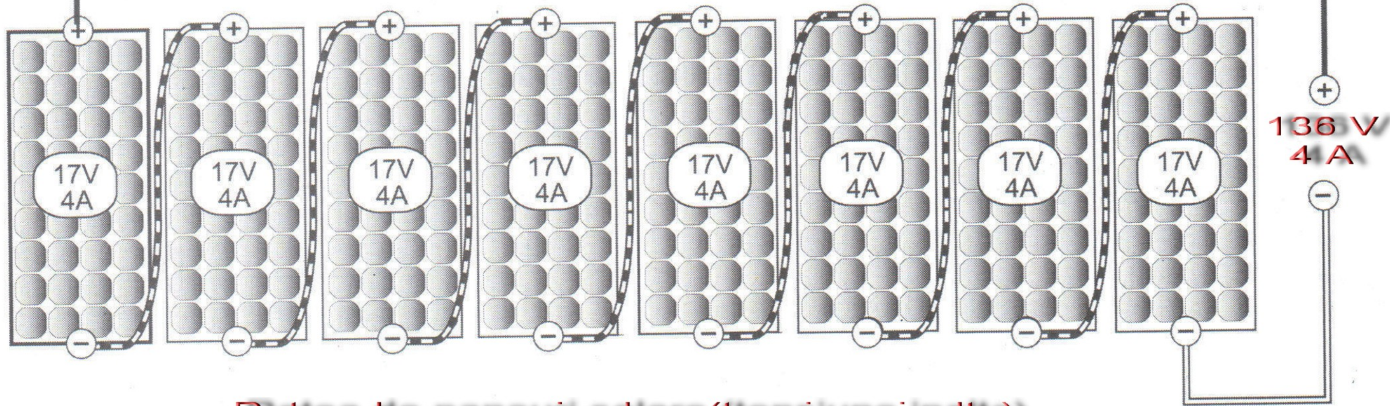
Retea de panouri solare (tensiune inalta)
